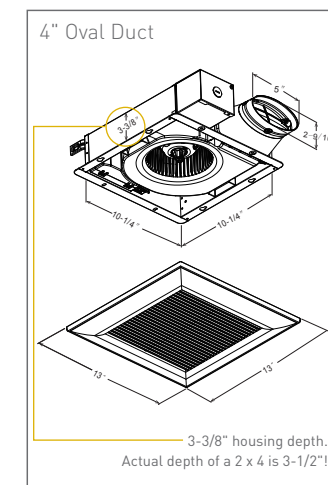
FV-0510VS1
