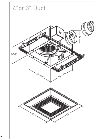
FV-0511VFL1
