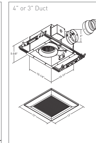
FV-0511VFC1
