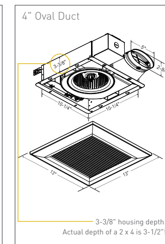
FV-0810VSS1
