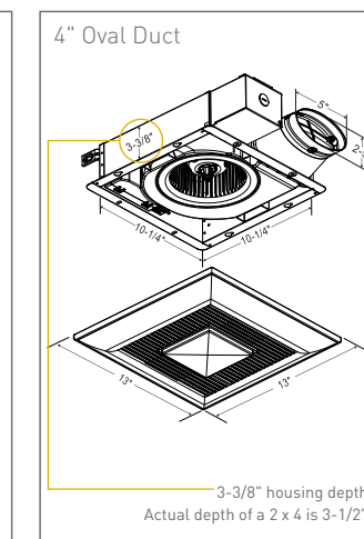
FV-0510VSL1
