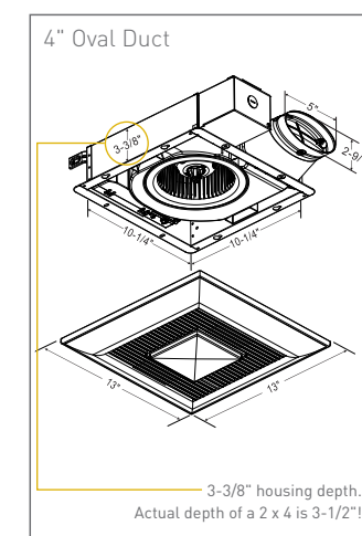
FV-0810VSSL1
