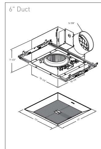
FV-1115VK3
