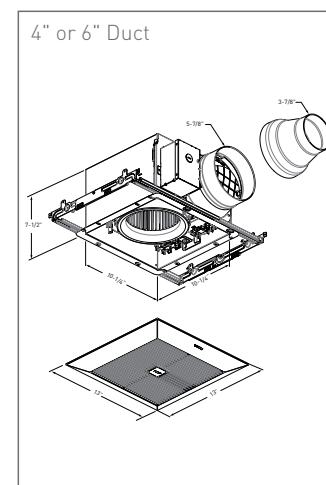
FV-0511VK3
