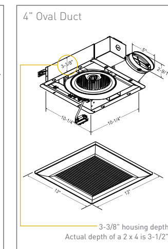
FV-0510VSC1
