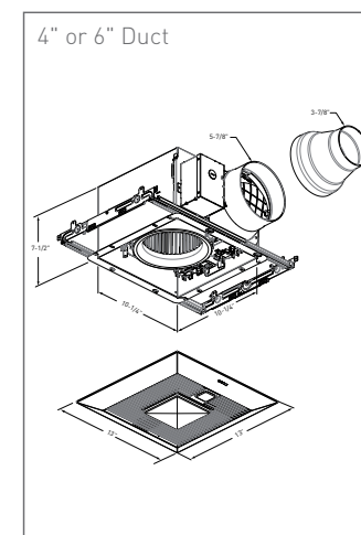
FV-0511VKL3
